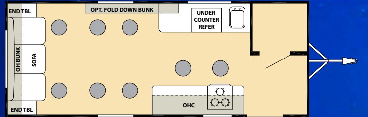
T8X20RC
