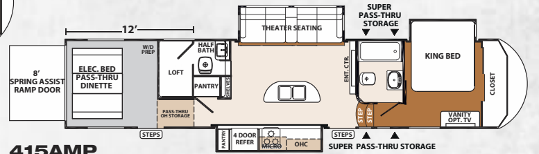
415AMP
