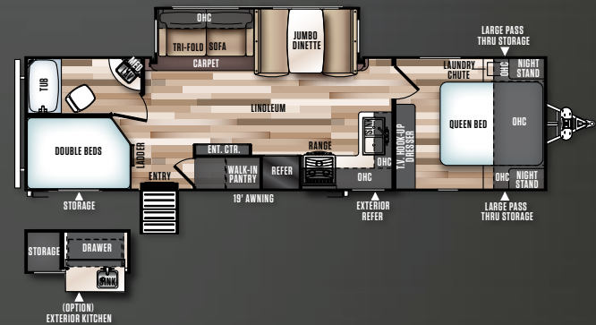
26BHKHL FLOORPLAN
