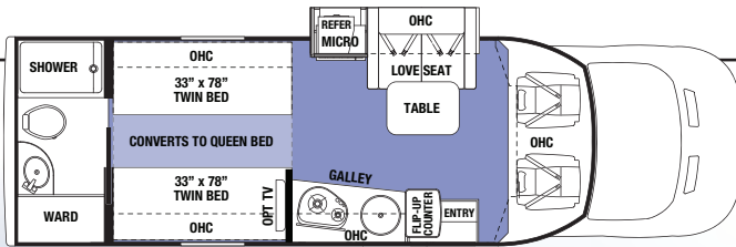
TS2370 (Moteur diesel seulement)
